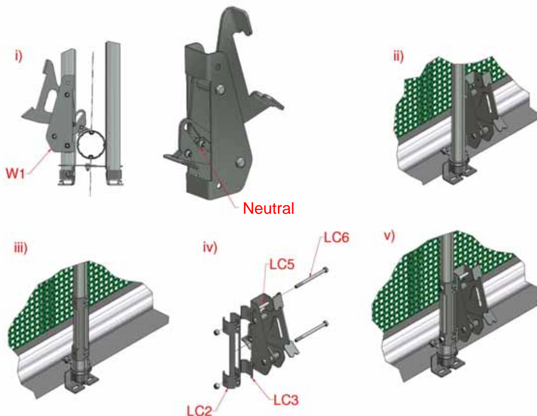
Figur 27, mellemliggende låsepaler
