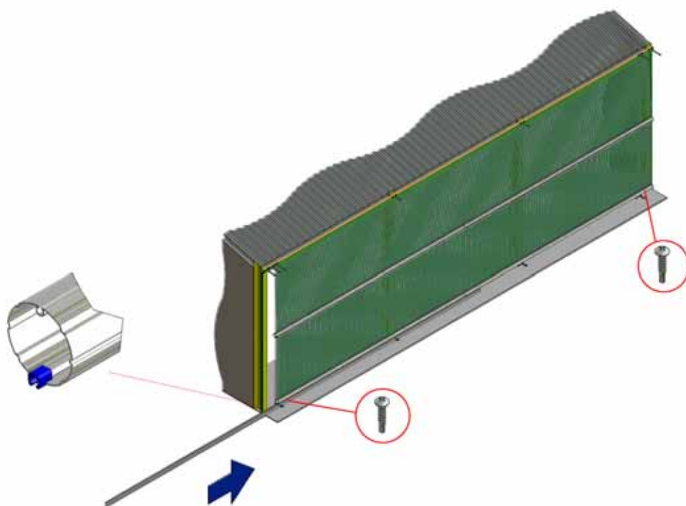
Figur 14, fastgørelse af den nederste flap
