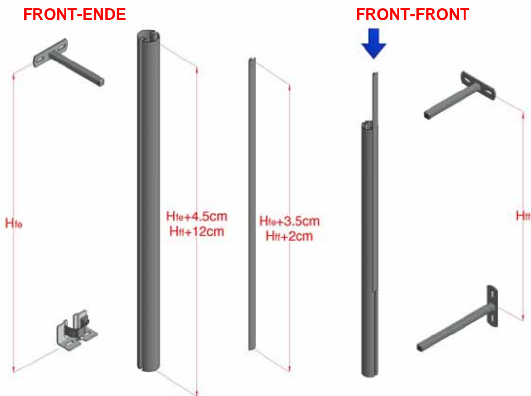
Figur 22, Udvendig kontrolslangesamling
