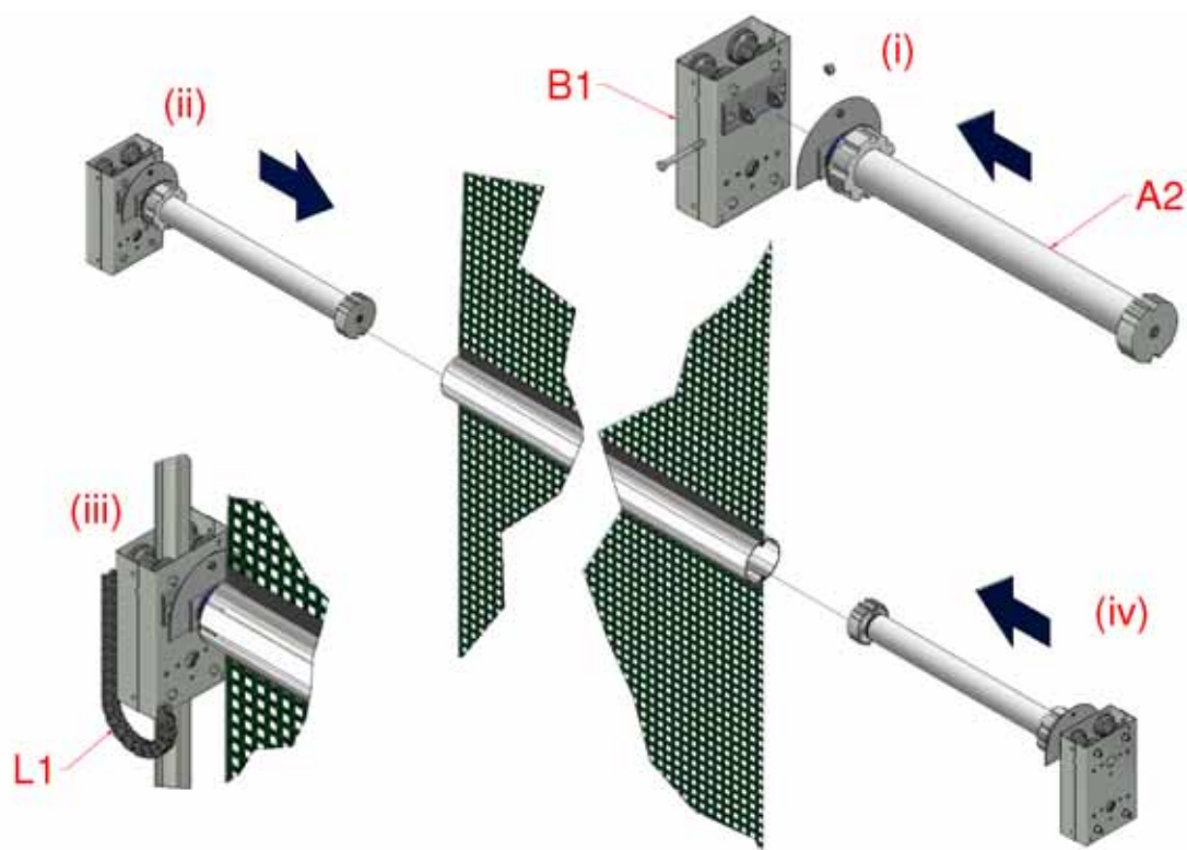
Figur 20, Dobbelt motor og vognboks
