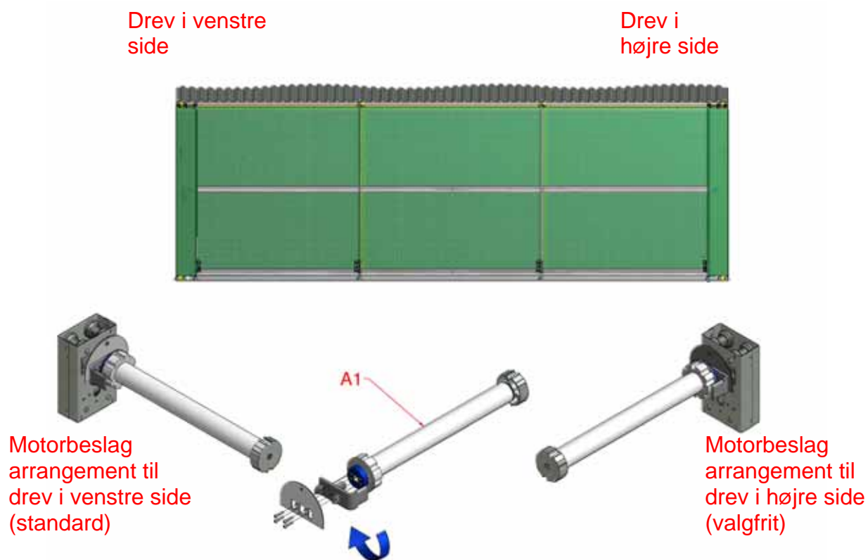
Figur 2b, muligheder for drevmotorende
