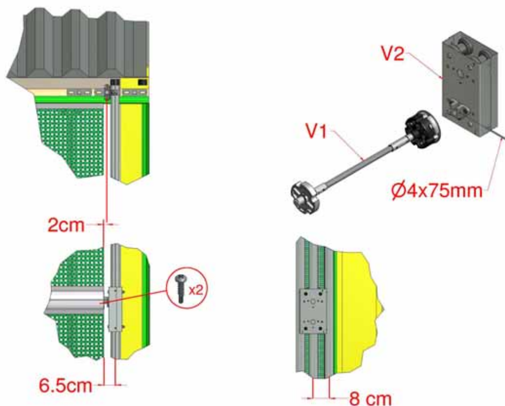
Figur 29, vognboks i den fri ende
