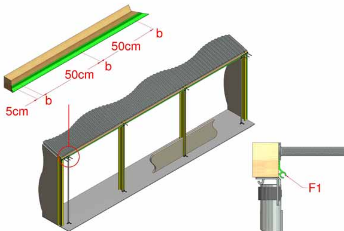
Figur 9, fastgørelse kador-profilen
