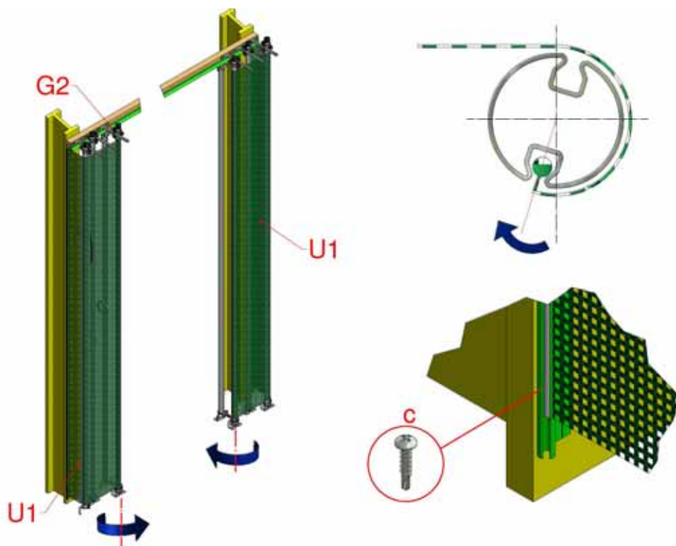
Figur 24, Endebeslag
