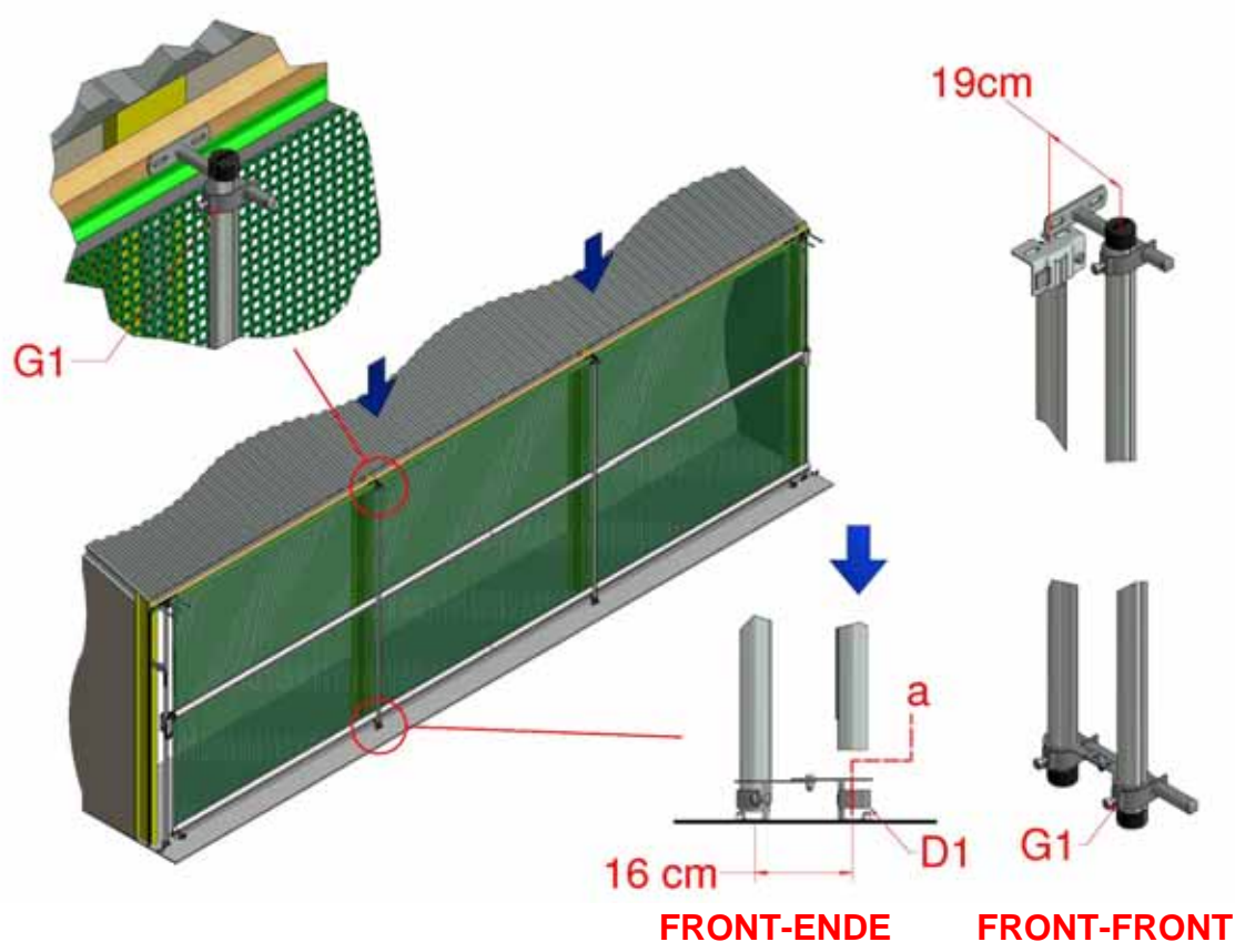
Figur 23, montering af ydre kontrolslange
