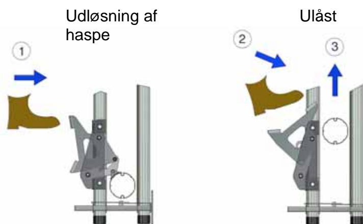
Figur 31, oplåsning af gardinet
