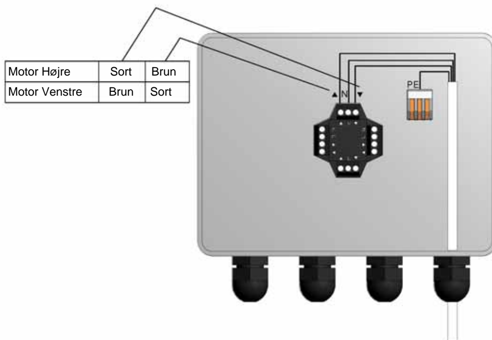
Figur 19, afbryderboksens ledninger
