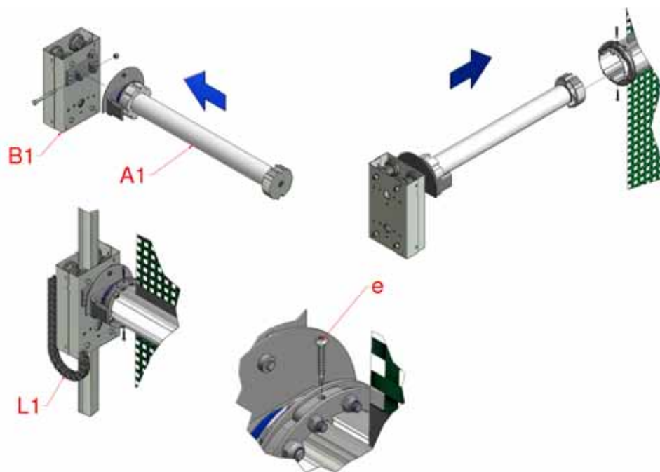
Figur 17, Enkelt motor og vognboks
