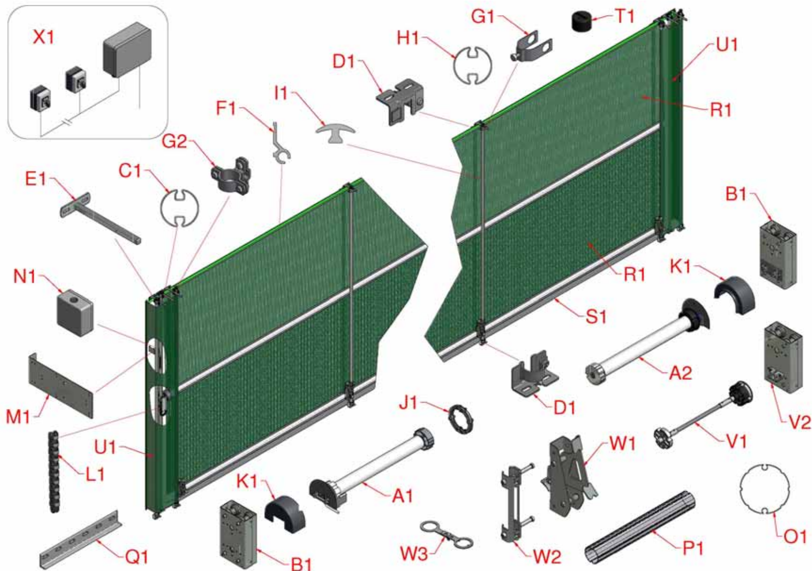
Figur 1, systemoversigt
