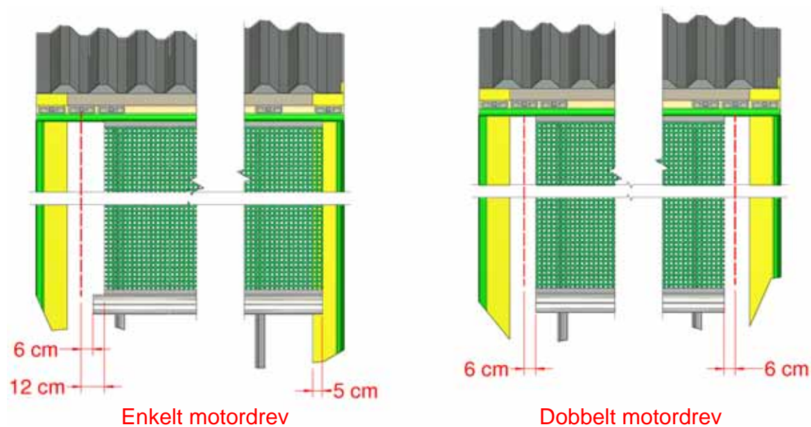
Figure 11b, Rørlængder
