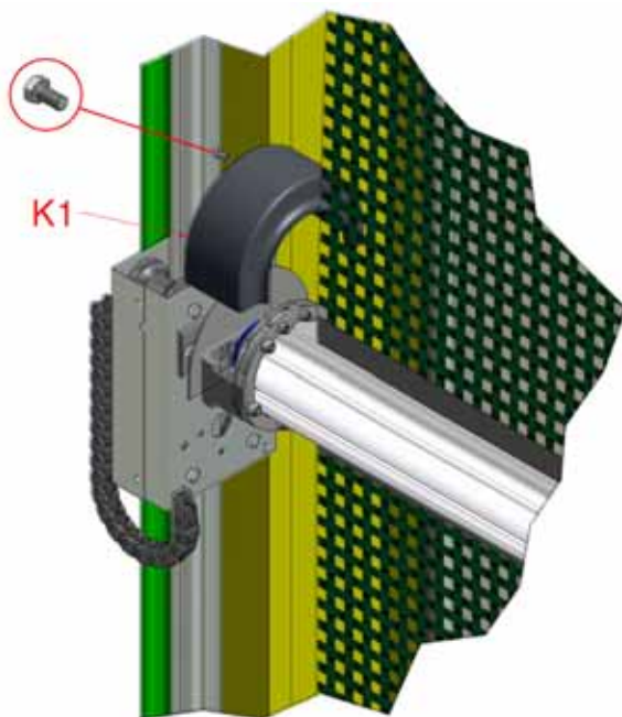
Figur 25, dæksel til vognboks
