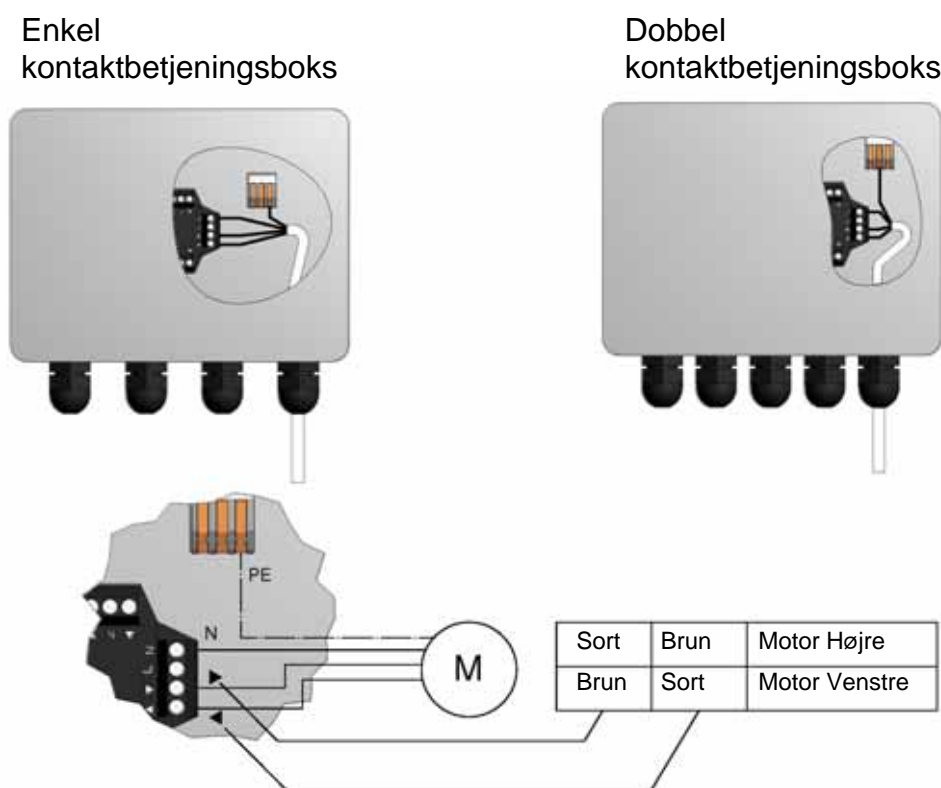
Figur 21, afbryderboksens ledninger
