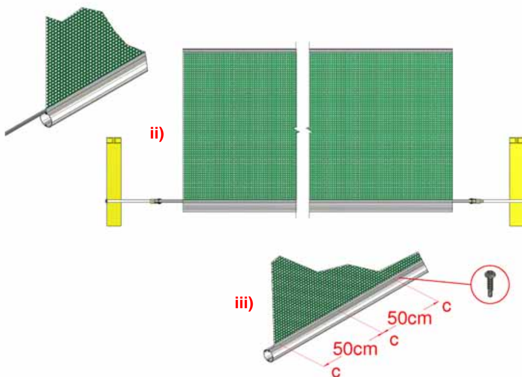
Figur 12, spændingsgardin
