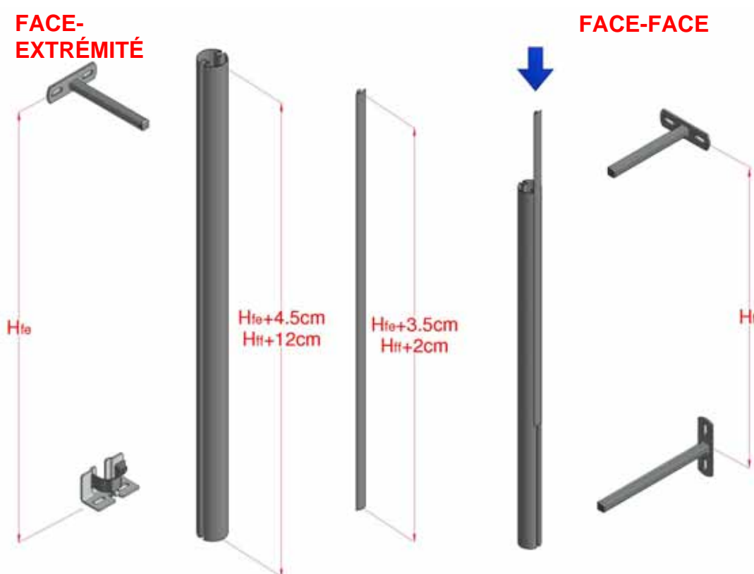
Figure 22 : montage du tube de commande extérieur
