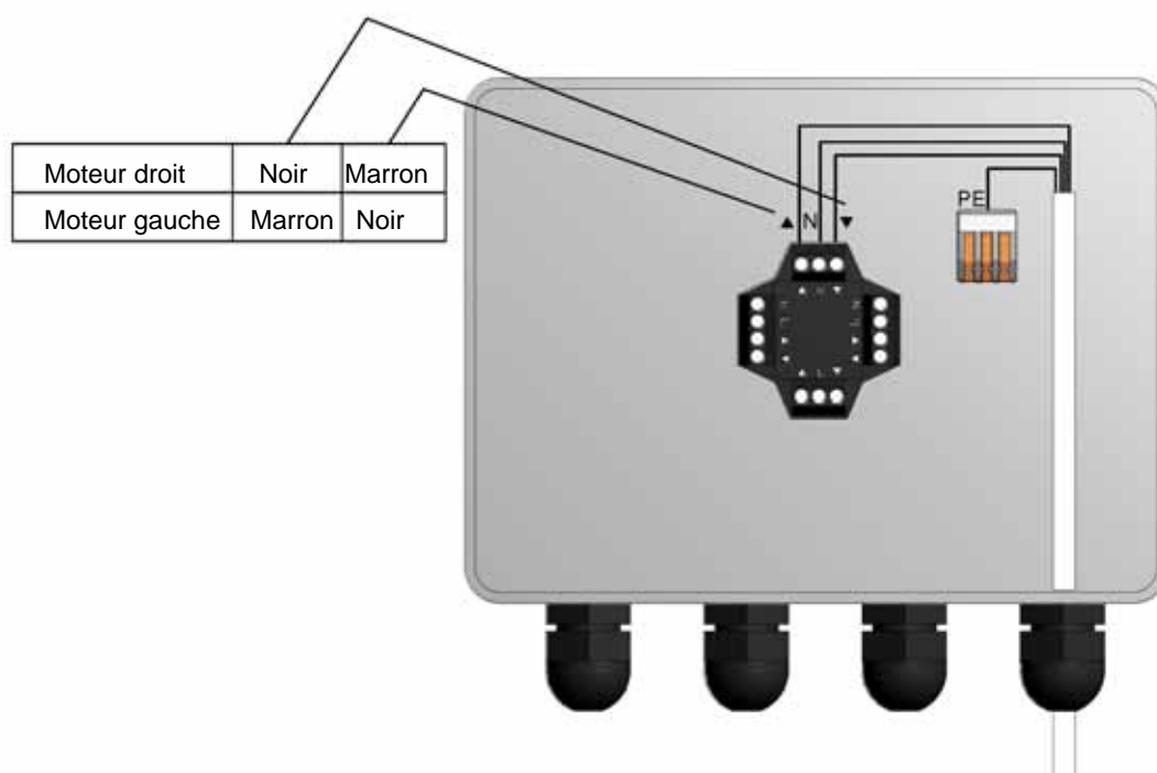
Figure 19 : câblage du boîtier de commande
