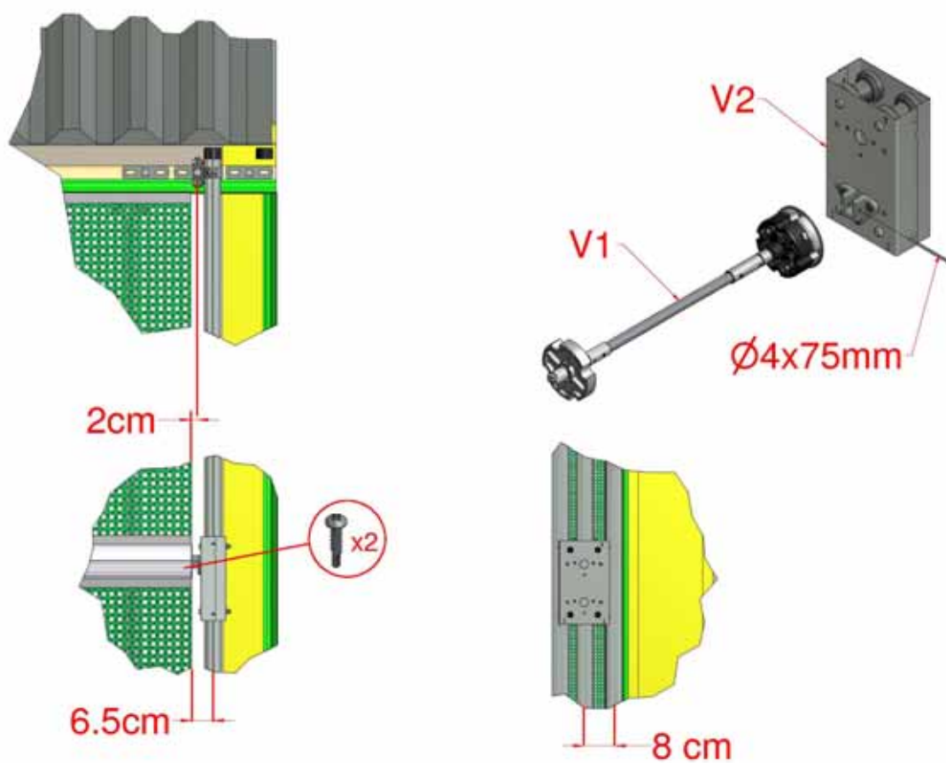
Figure 29 : coffret de commande d'extrémité libre
