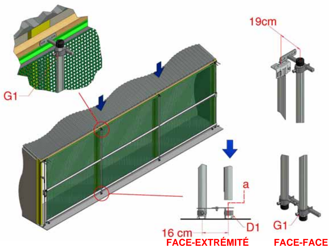
Figure 23 : pose du tube de commande extérieur
