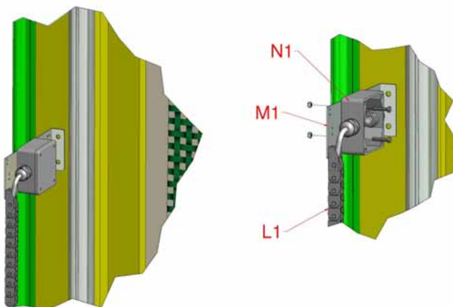
Figure 18 : montage de la boîte de raccordement
