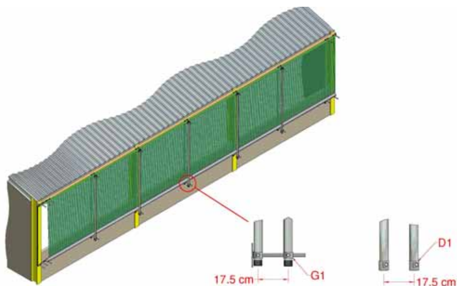
Afbeelding V4, Buitenste stuurbuizen
