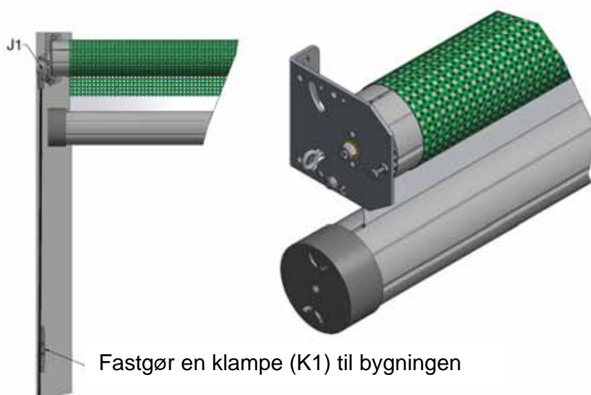
Figur 8, Klampe
