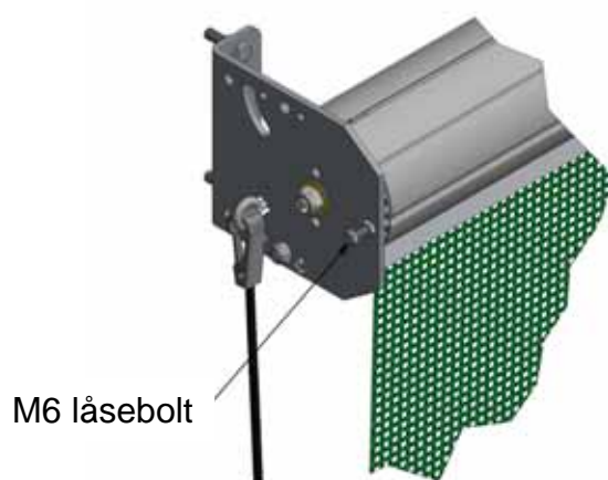
Figur 11a, Låsebolt
