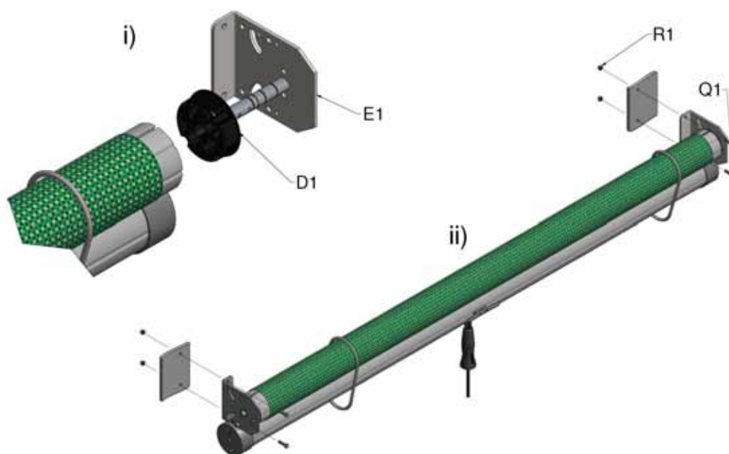
Figur 7a, Montering af skærme op til en bredde på 5,0 m på en bygning
