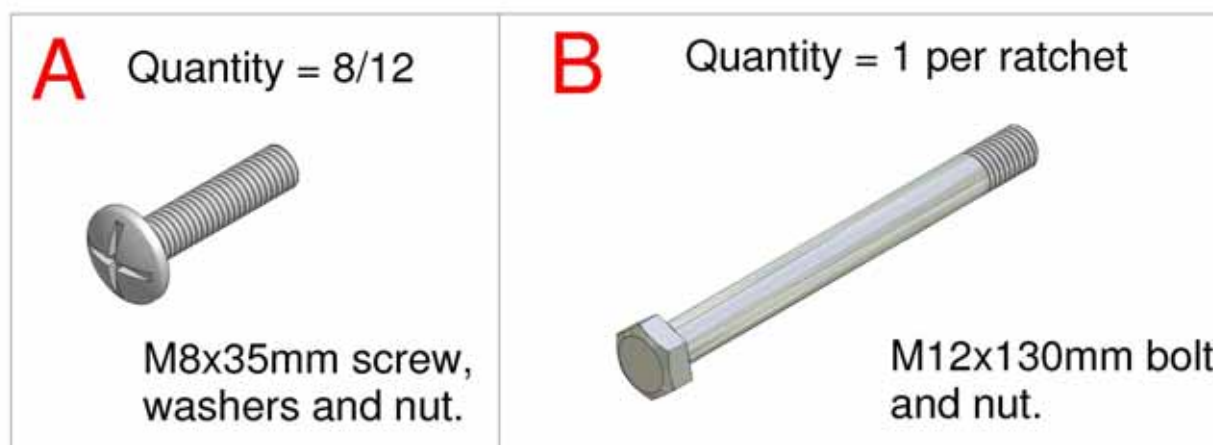
Afbeelding 2, Bevestigingsmiddelen en hoeveelheden
