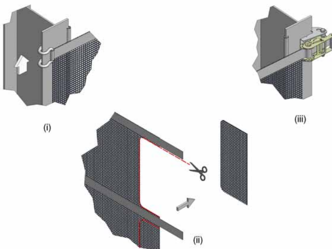
Afbeelding 5, montage van het scherm
