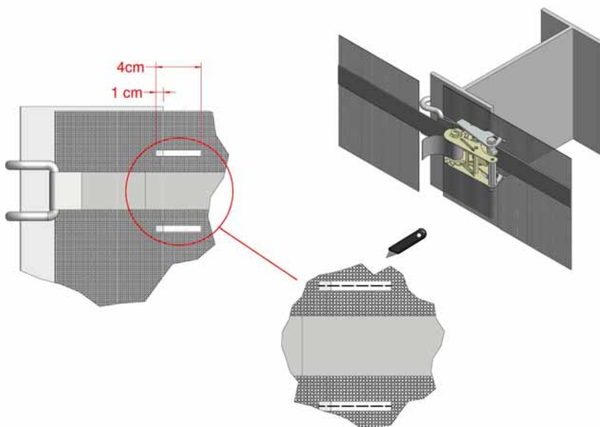
Afbeelding 8, schermen naast elkaar monteren
