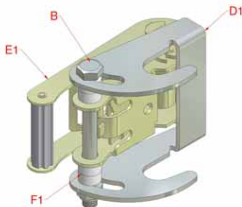
Afbeelding 6, 50 mm haak- en palmontage
