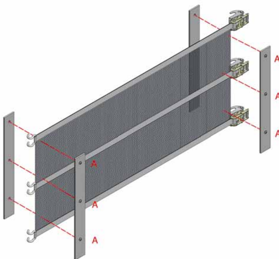
Afbeelding 9, De eindbuffers bevestigen
