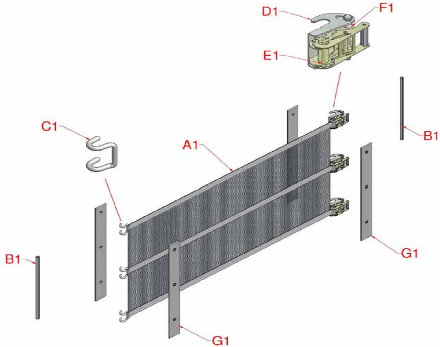
Afbeelding 1, Systemoverzicht en afzonderlijke componenten
