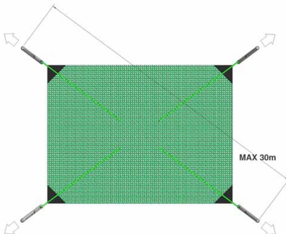
Figuur 3, Opstelling van de palen
