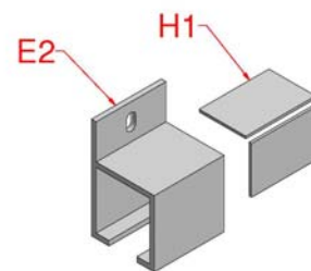
Figur 5, Skinnefastgørelse
