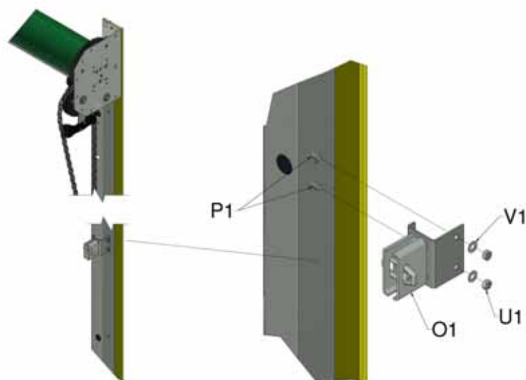
Figure 13, fixer le guide-chaîne au rail de guidage
