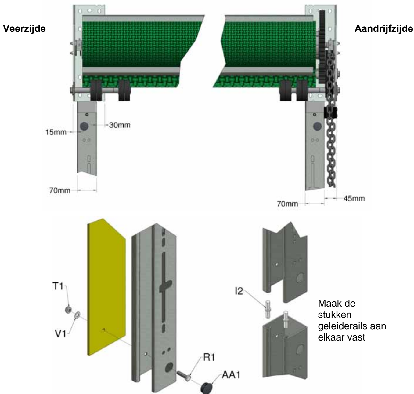
Afbeelding 11, Bevestiging van geleiderail aan de muur en de verbinding van de geleiderail
