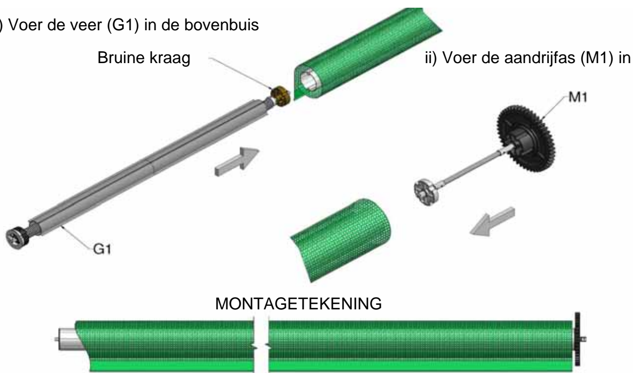
Afbeelding 6c, Bovenbuis (rechtse aandrijving)
