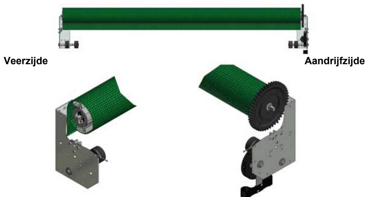
Afbeelding 7, Bovenbuis in bevestigingen plaatsen (rechtse aandrijving getoond)
