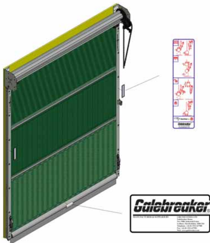
Afbeelding 18, Bevestigen van labels
