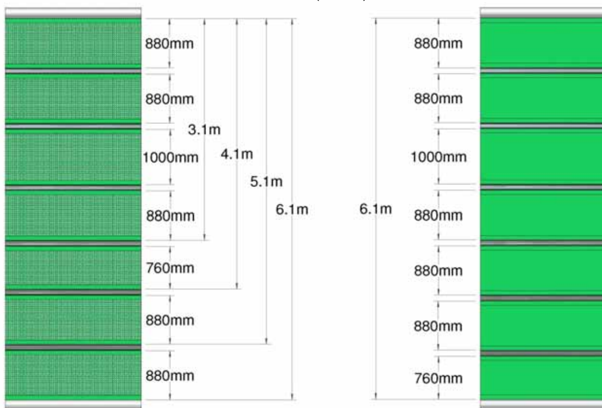
Afbeelding 5b, Ventilatiepaneel-layout
