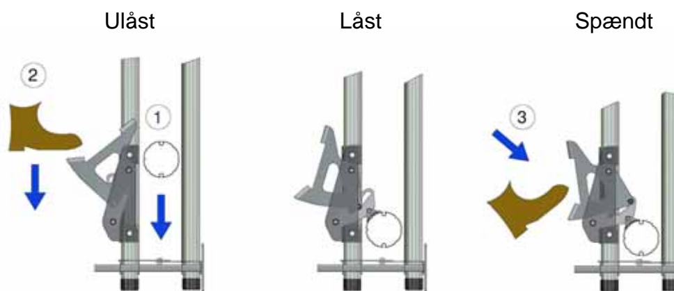
Figur 28, låsning af gardinet
