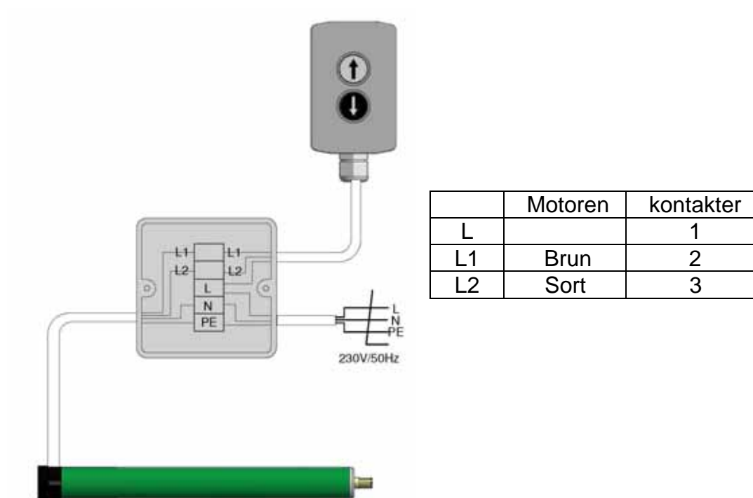
Figur 21a, Motor Venstre
