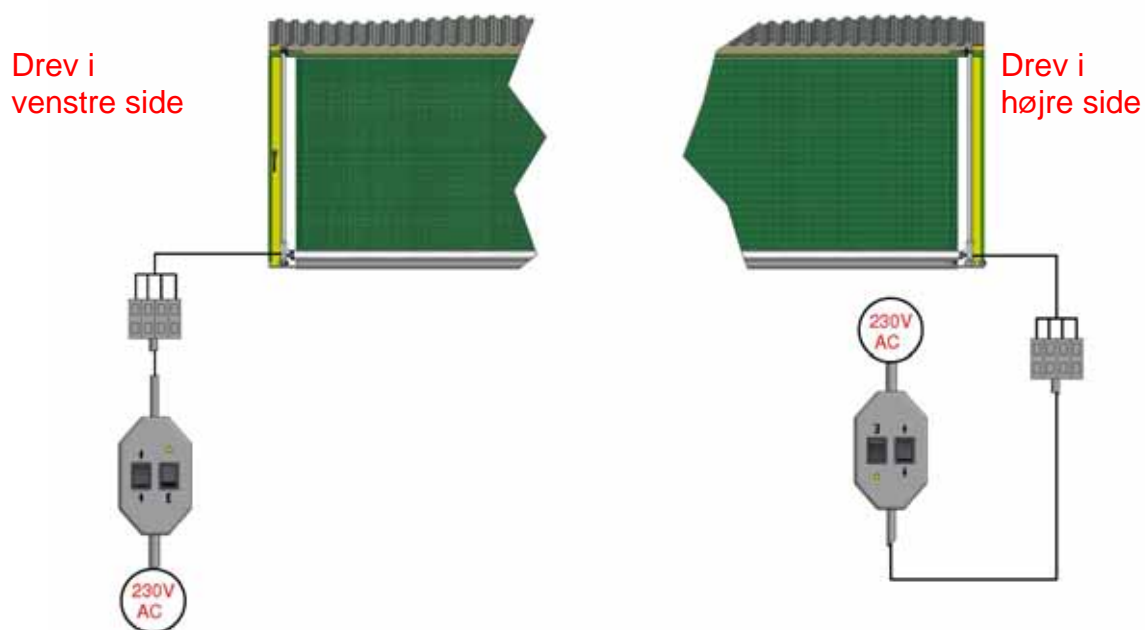
Figur 17a, indstillingskontakten
