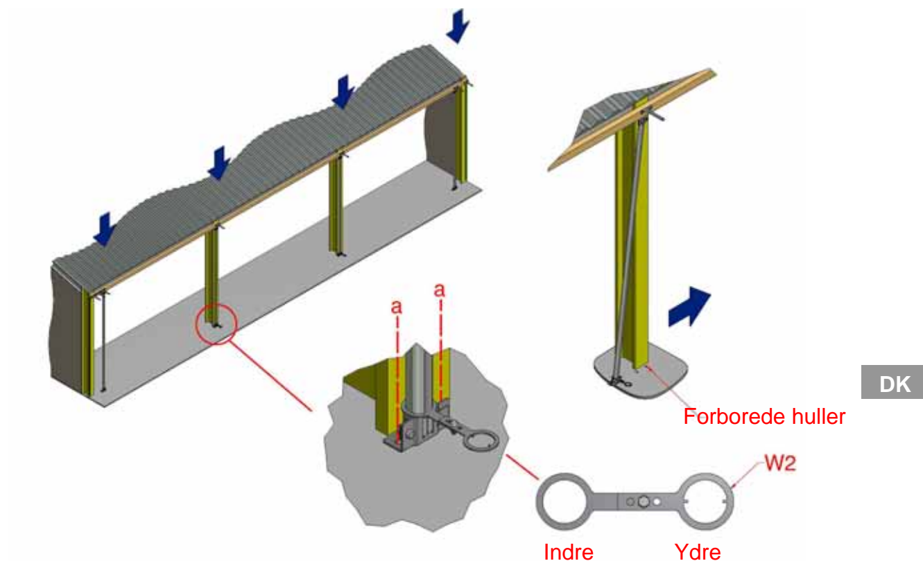
Figur 7, indvendige kontrolslanger front-ende
