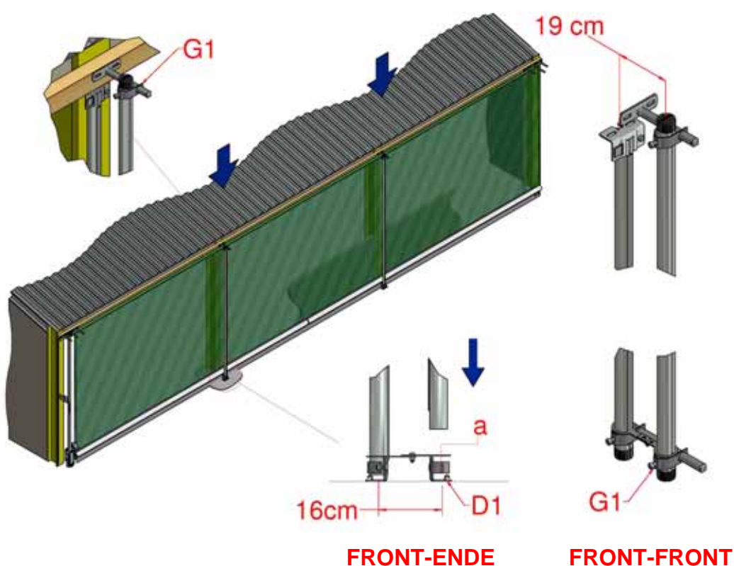
Figur 19, montering af ydre kontrolslange
