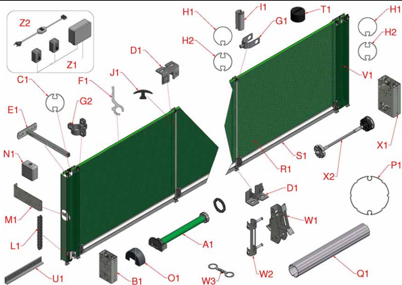
Figur 1, systemoversigt
