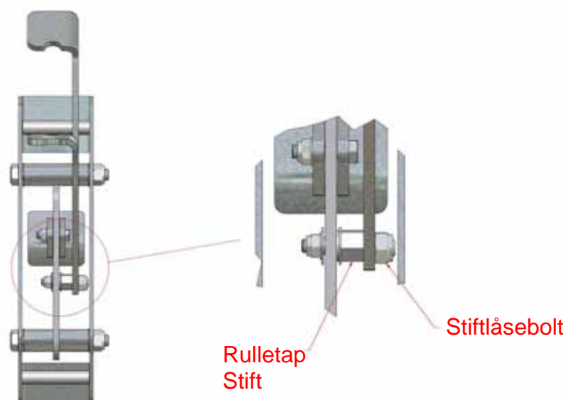
Figur 31, justering af låsehakker
