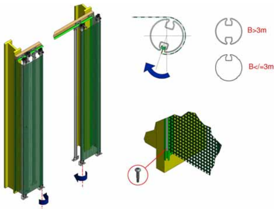
Figur 22, Endebeslag
