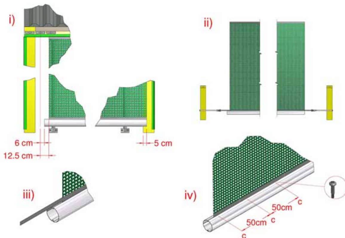
Figur 12, spændingsgardin
