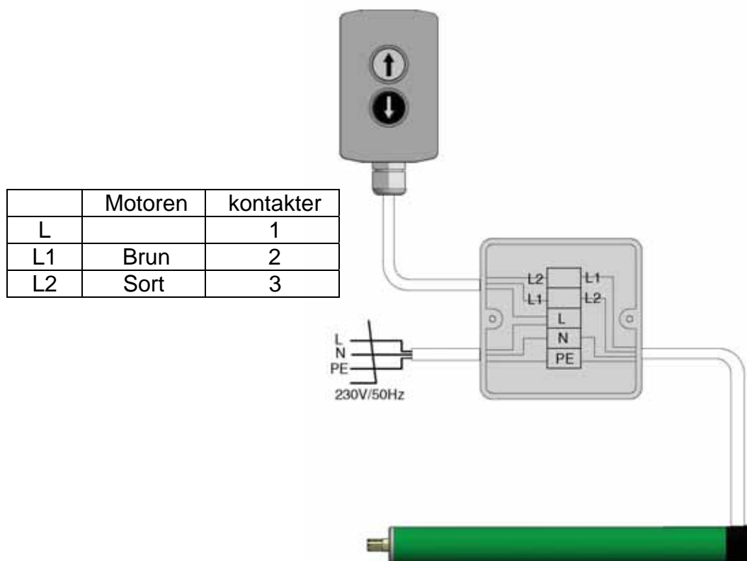
Figur 21a, Motor Højre
