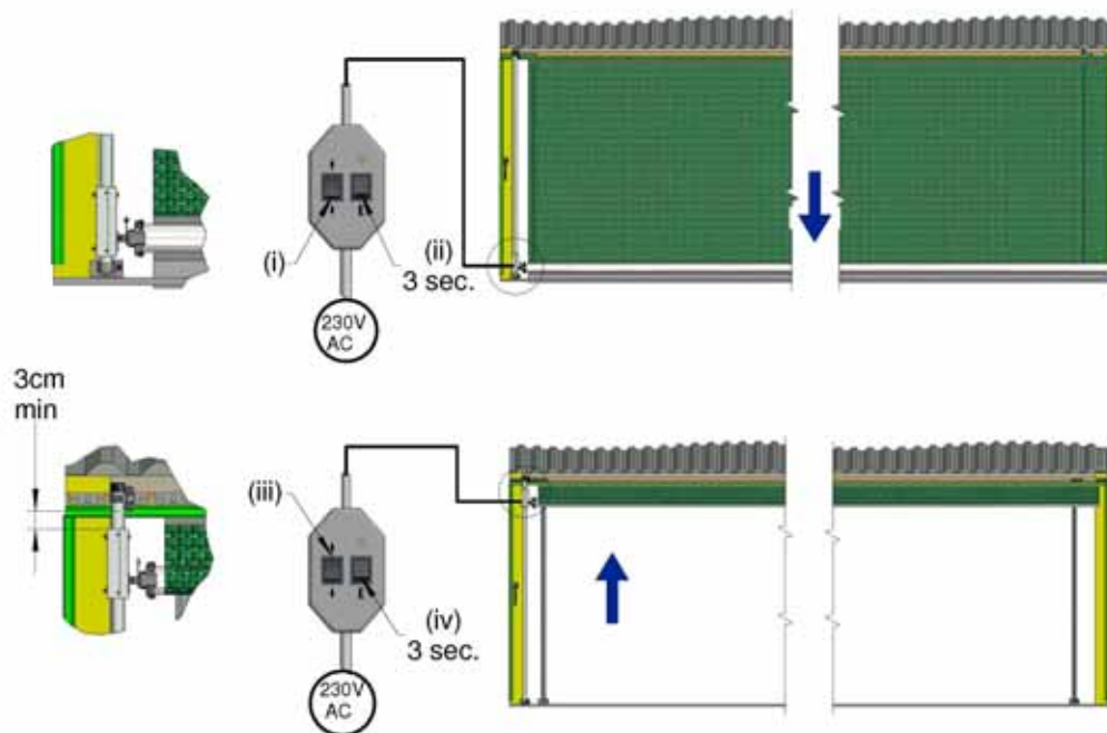
Figur 20a, Indstilling af grænserne (i)
