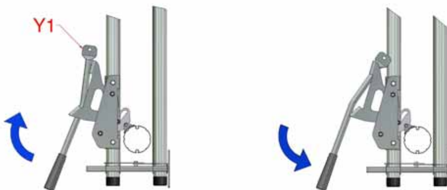
Figur 30, manuel betjening af låsepal
