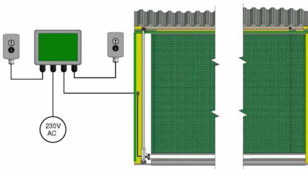
Figur 17b, afbryderboksens ledninger
