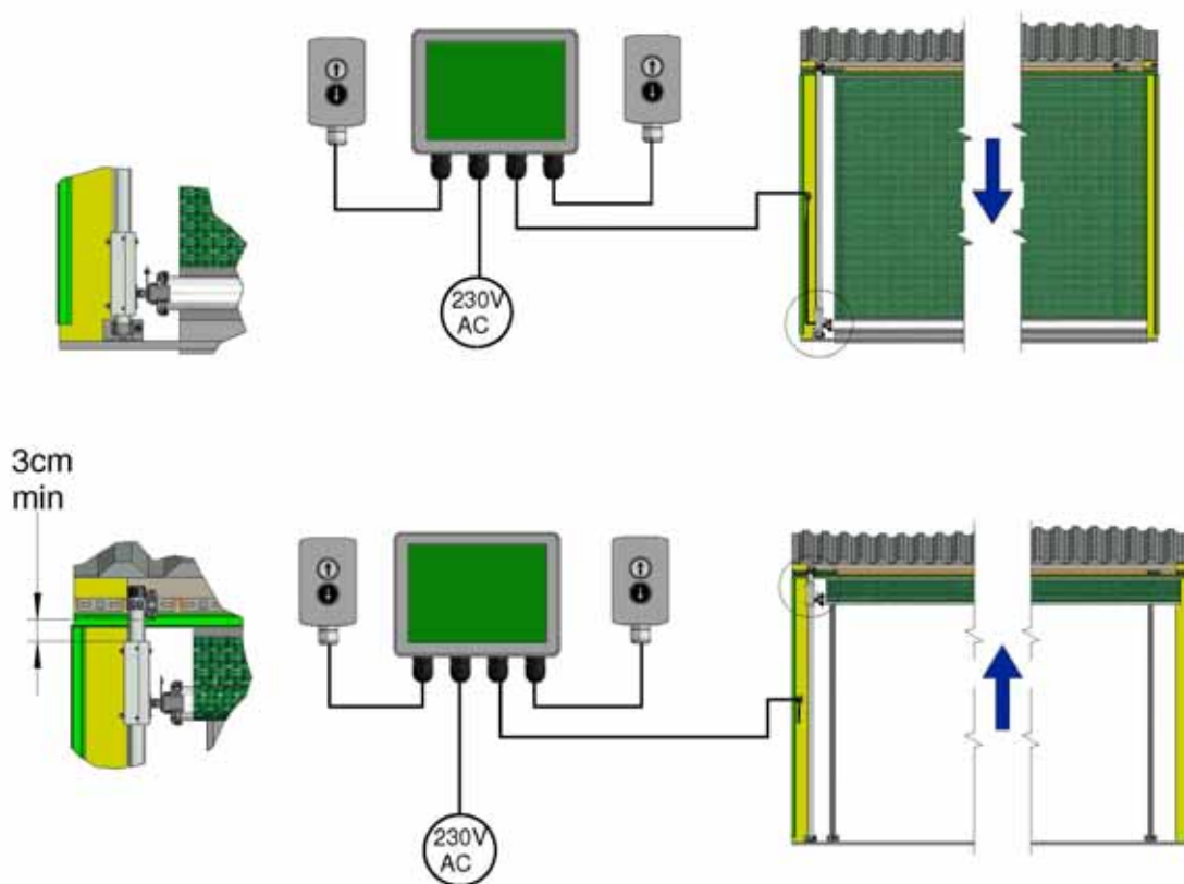
Figur 20b, Indstilling af grænserne (ii)
