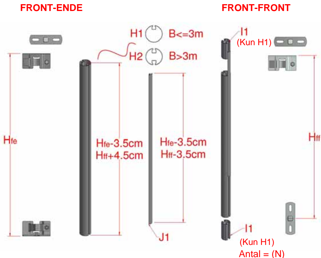
Figur 6, indvendig kontrolslangesamling
