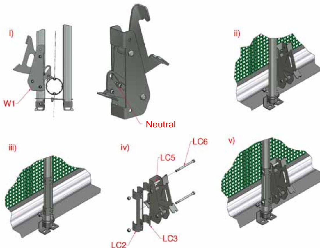
Figur 25, mellemliggende låsepaler
