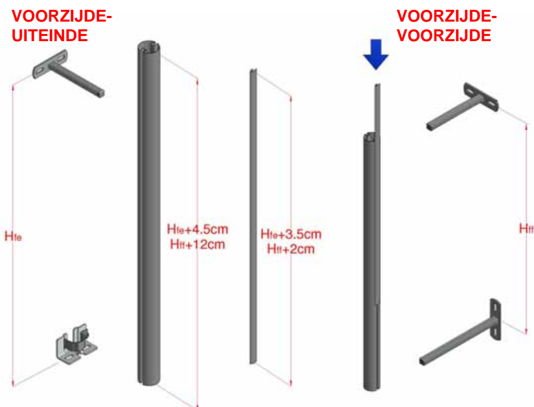
Afbeelding 20, Montage buitenste stuurbuizen
