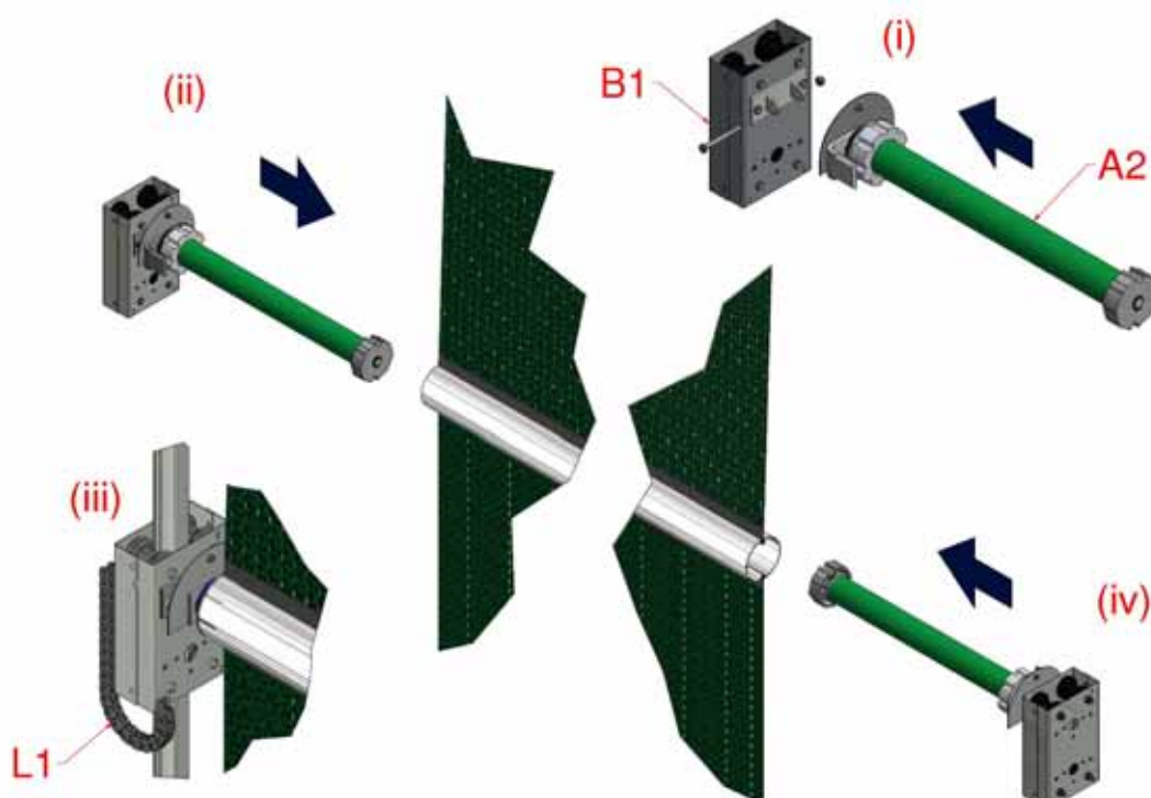
Afbeelding 24, Dubbele motor en katrolkast
