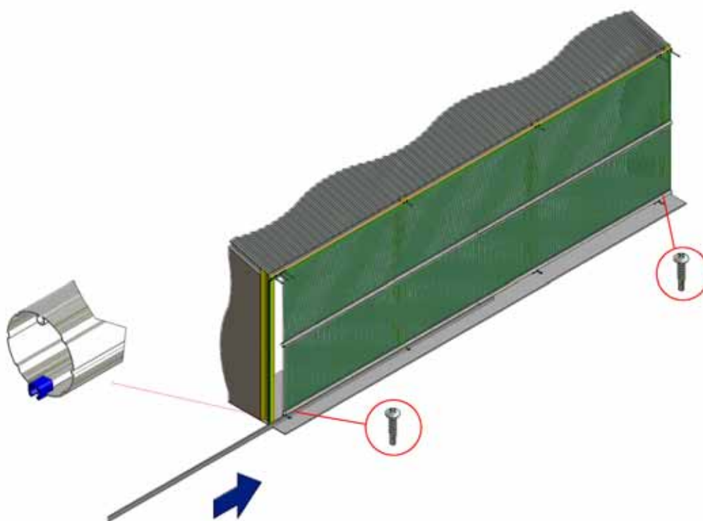
Afbeelding 14, De benedenflap bevestigen
