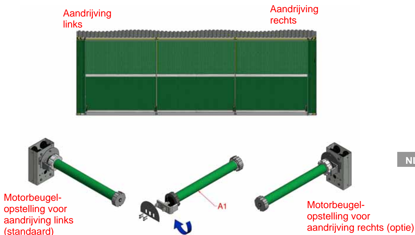
Afbeelding 2b, Opties voor zijde met aandrijfmotor
