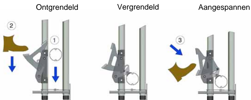
Afbeelding 31, Het scherm vergrendelen
