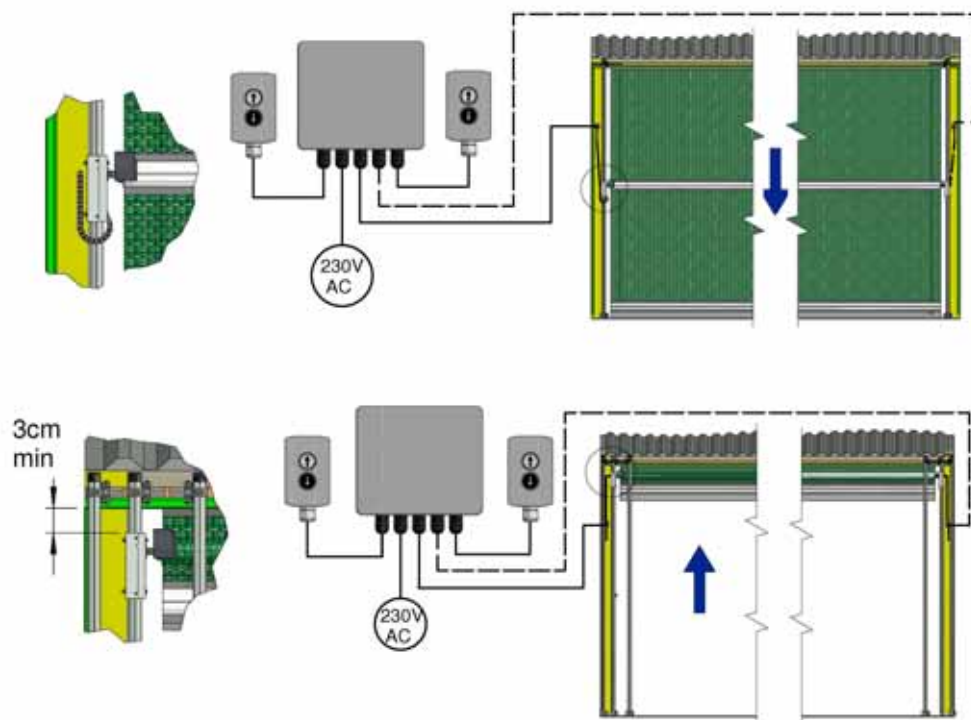
Afbeelding 22b, De begrenzingen instellen (ii)
