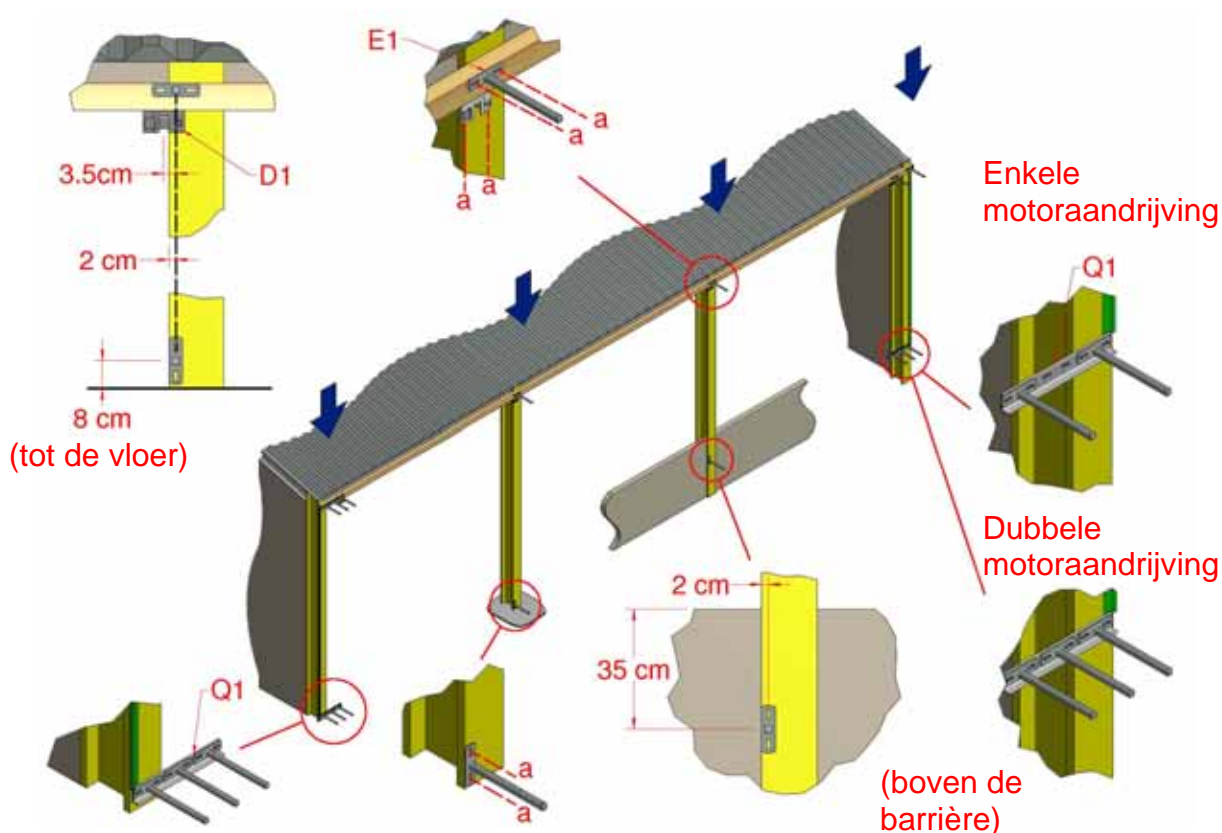
Afbeelding 5b, Installatie van tussenliggende stuurbuisbeugels (voorzijde-voorzijde)
