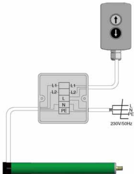
Afbeelding 23a, Motor links
