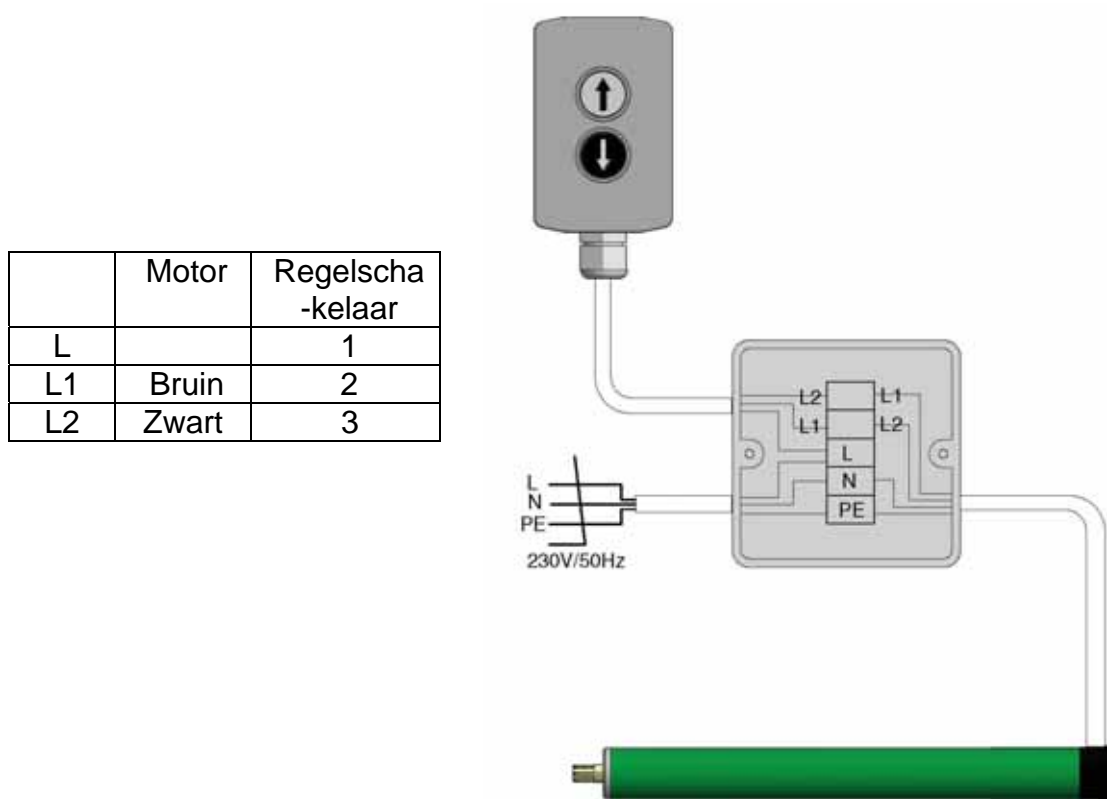
Afbeelding 23b, Motor Rechts
