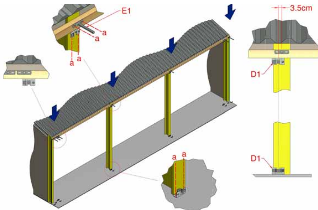
Afbeelding 5a, Installatie van tussenliggende stuurbuisbeugels (voorzijde-uiteinde)
