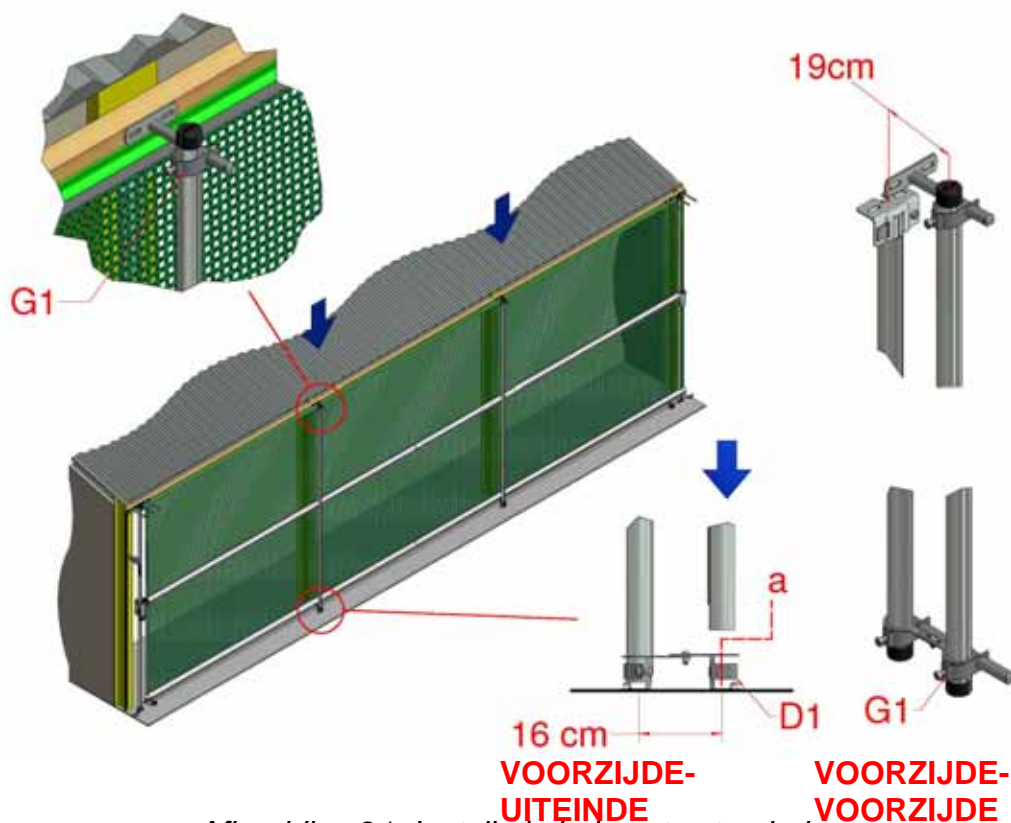
Afbeelding 21, Installatie buitenste stuurbuizen
