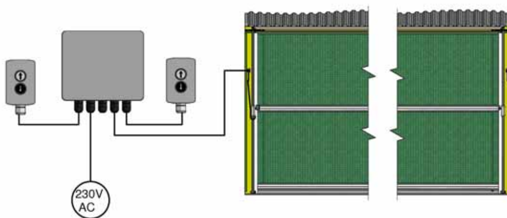
Afbeelding 19b, Bedrading schakeldoos
