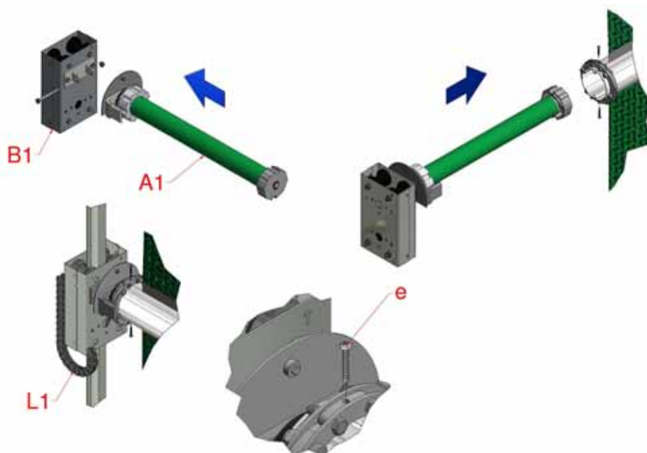
Afbeelding 17, Enkele motor en katrolkastje
