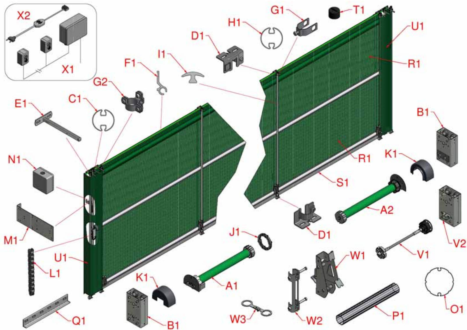
Afbeelding 1, Overzicht van het systeem
