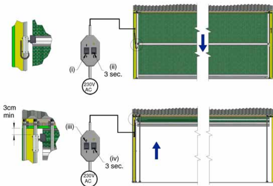
Afbeelding 22a, De begrenzingen instellen (i)
