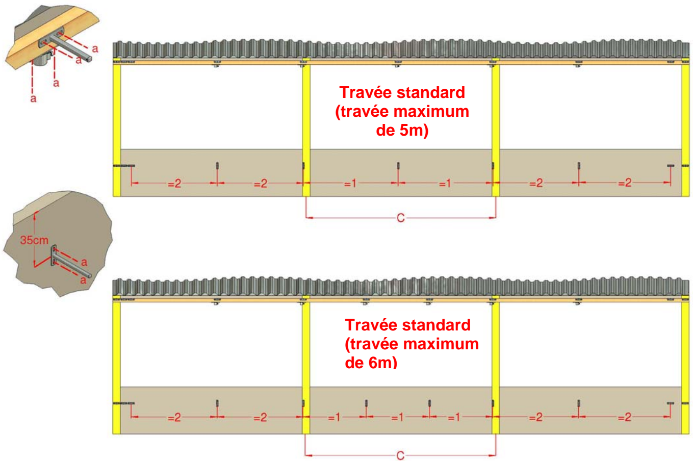
Figure V2a : supports supplémentaires (Face-Face)
