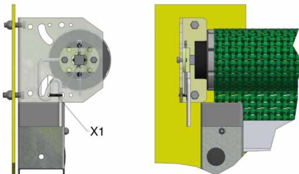
Figure 12, Fastgøring af motorledning
