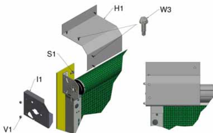
Figur 18, Montering af motorskærm
