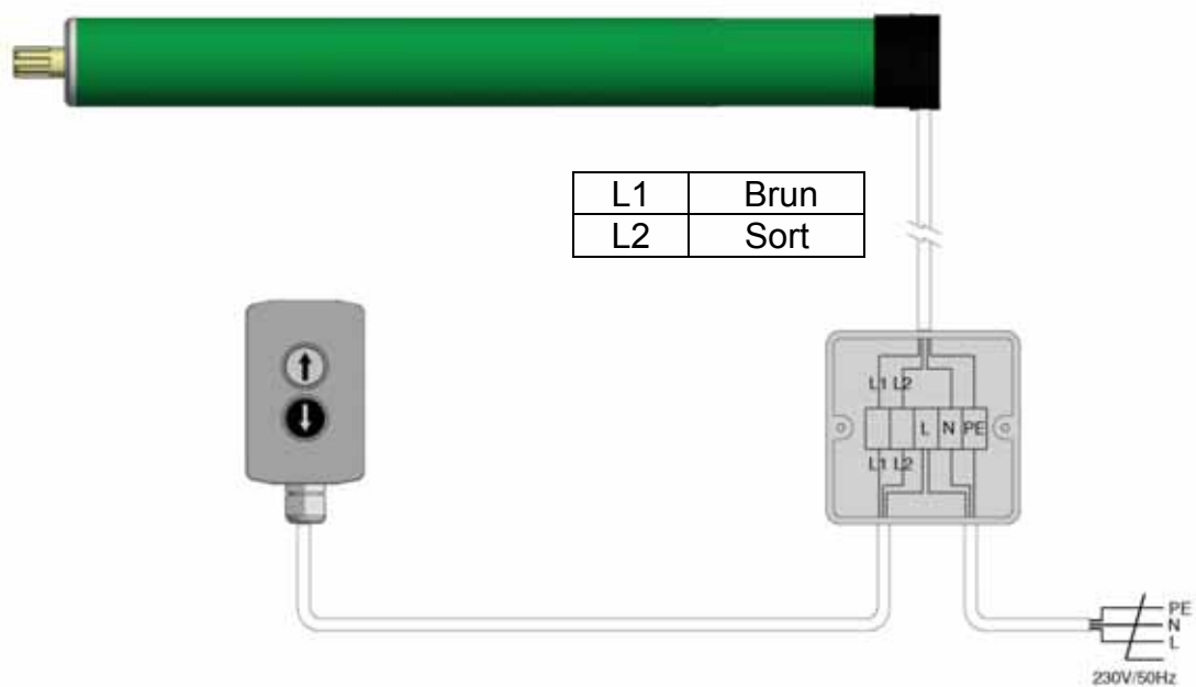
Figur 13a, Betjening med højre hånd
