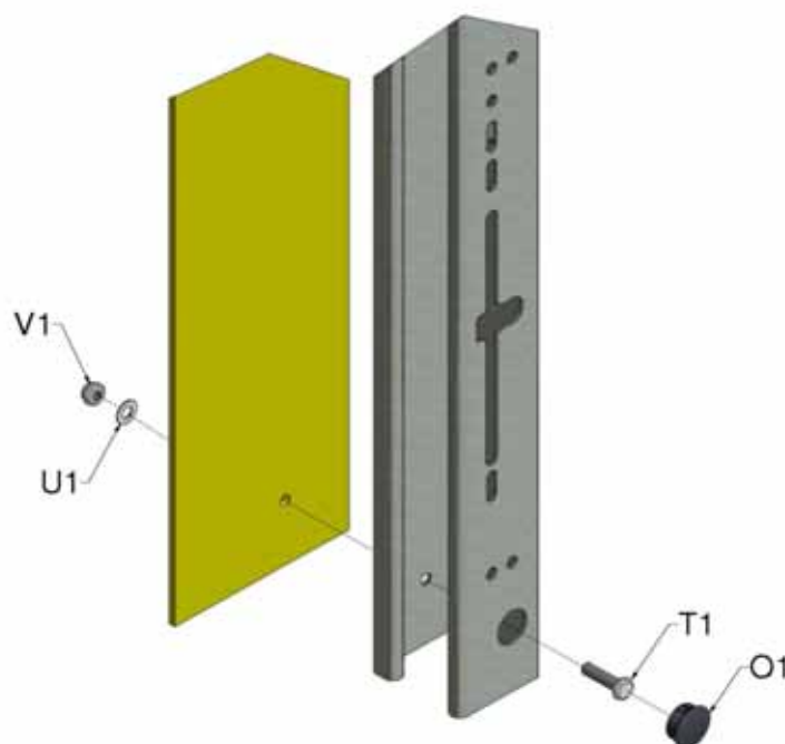
Figur 9b, Fastboltning af styreskinnen til væggen.
