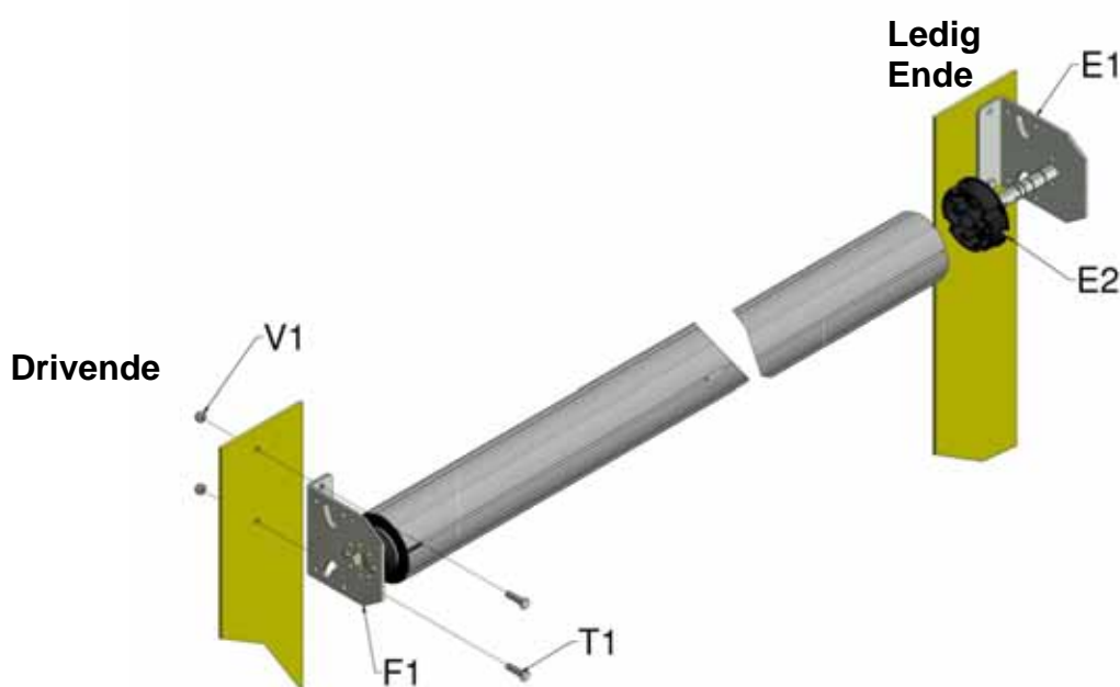
Figur 7a, Montering af døre op til en bredde på 5,0m på en bygning
