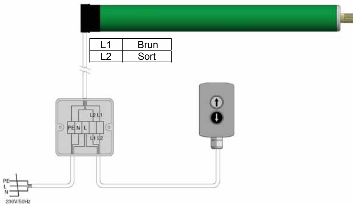
Figur 13b, Betjening med venstre hånd
