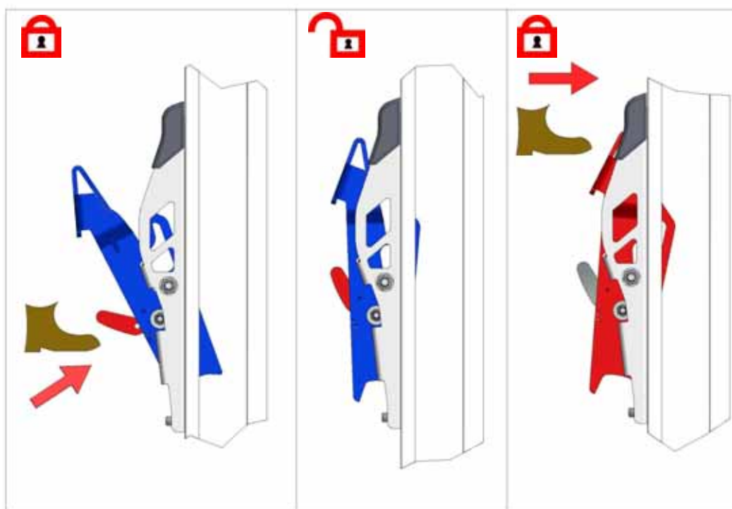
Figur 21, Aktivering og deaktivering af låsehagen
