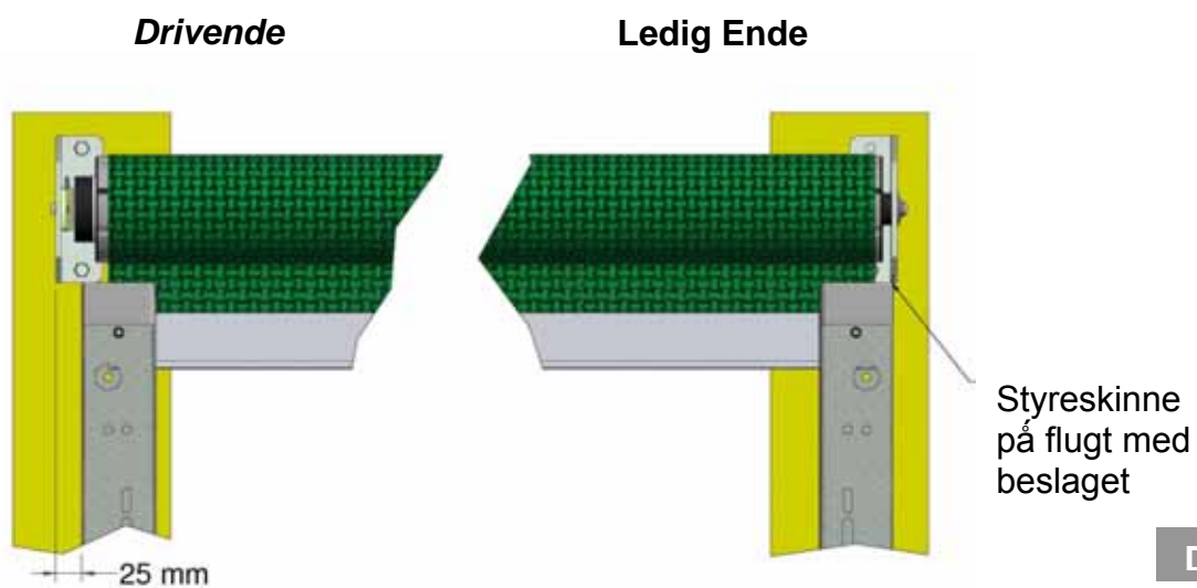
Figur 9a, Styreskinnens placering
