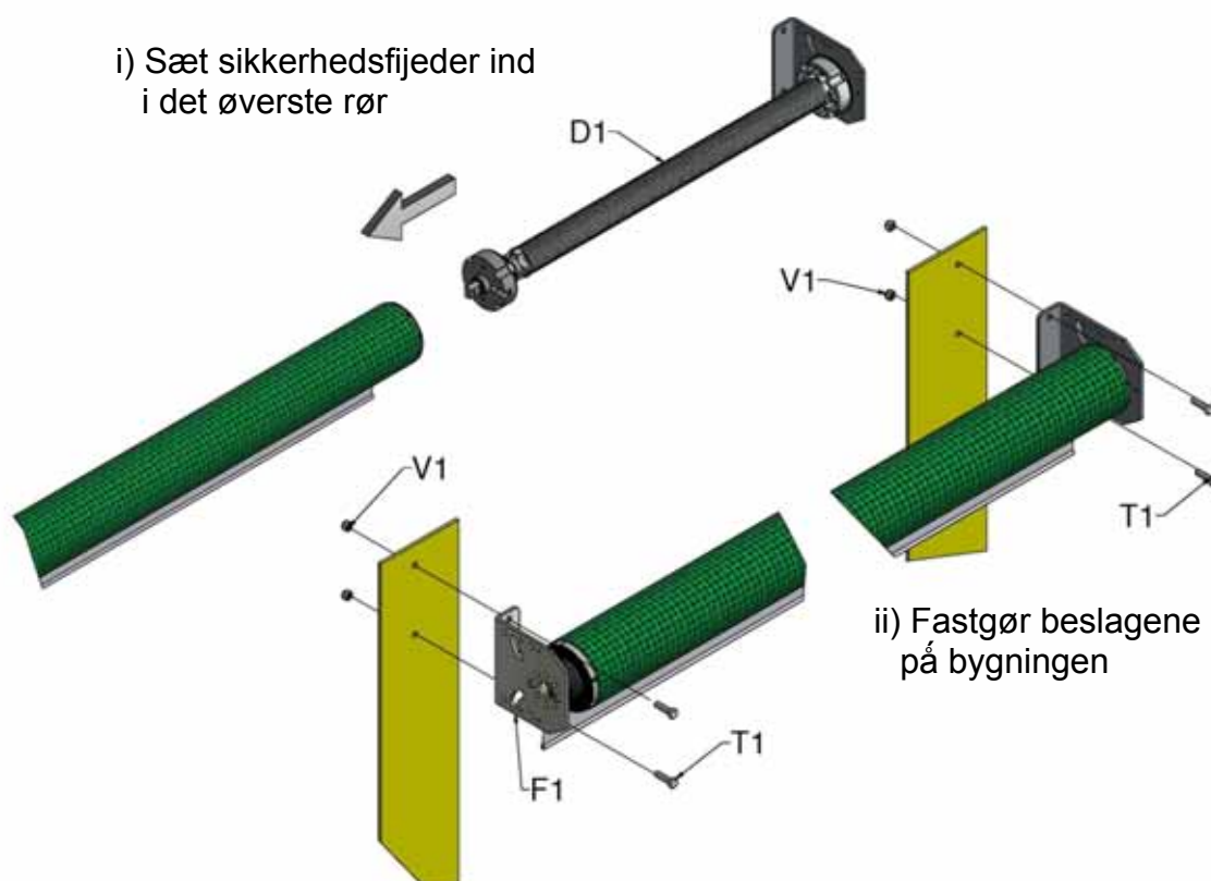
Figur 7b, Montering af døre med en bredde over 5,5m på en bygning
