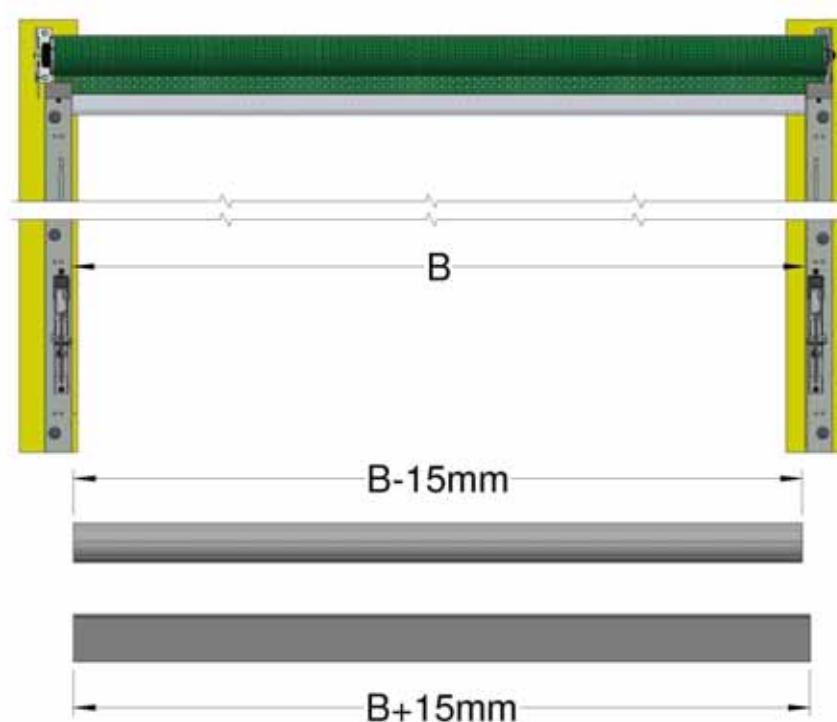
Figur 11, Sådan skæres nederste rørs længde, indsats og klap
