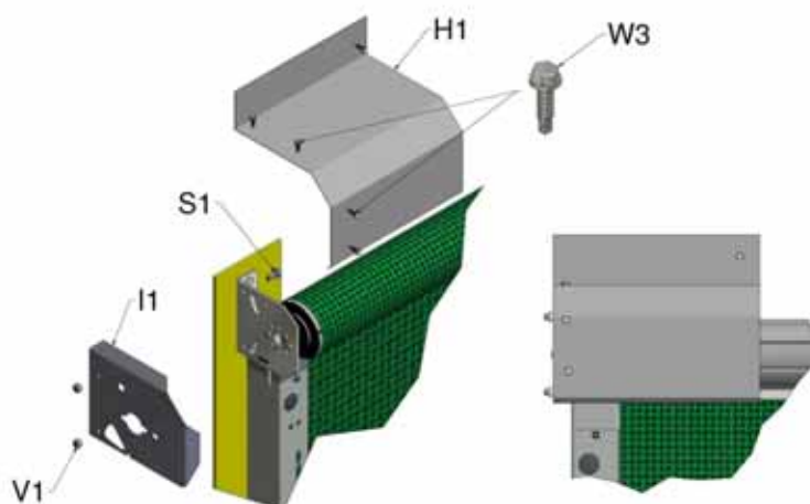
Figure 18, Ensemble du carénage du moteur
