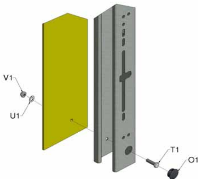
Figure 9b, Boulonnage du rail de guidage au mur.
