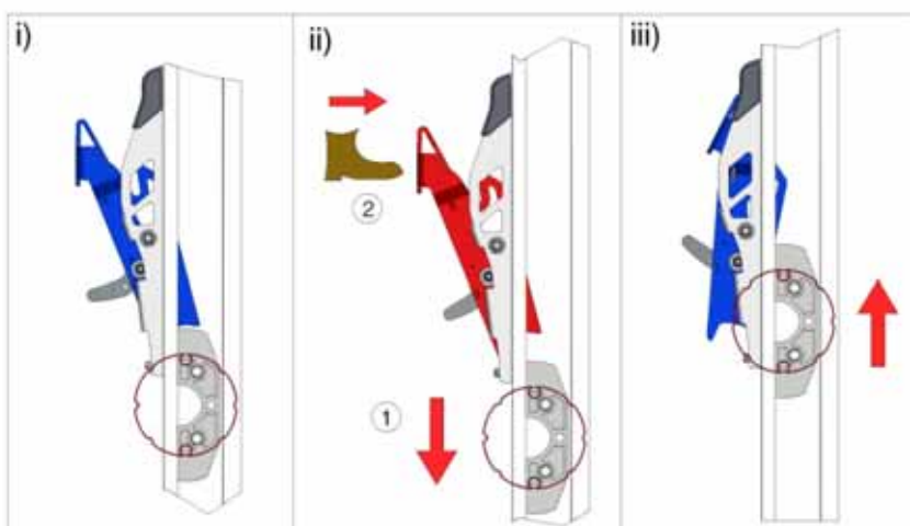
Figure 23, Ouvrir la porte depuis la position verrouillée
