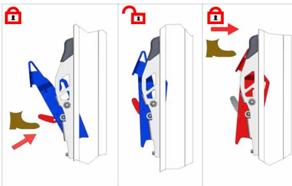
Figure 21, Embrayer et débrayer le cliquet de verrouillage
