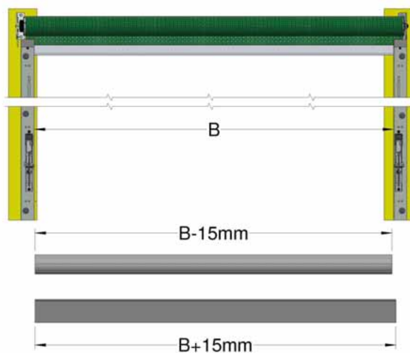
Figure 11, Couper la longueur du tube inférieur, de l'insertion et du rabat
