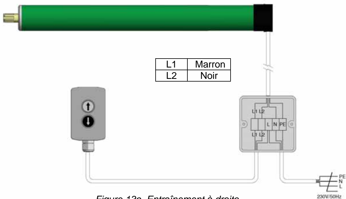
Figure 13a, Entraînement à droite
