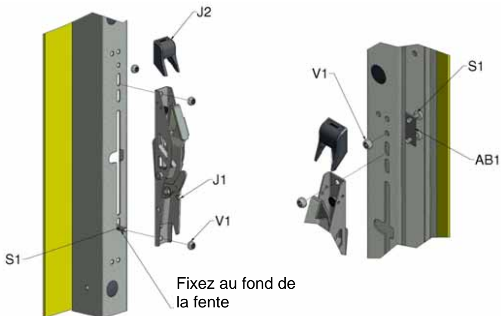
Figure 10, Boulonnage des cliquets de verrouillage
