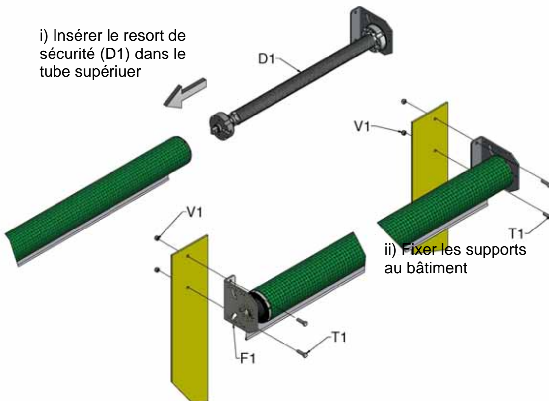
Figure 7b, Fixer les portes de plus de 5,5 m de largeur au bâtiment
