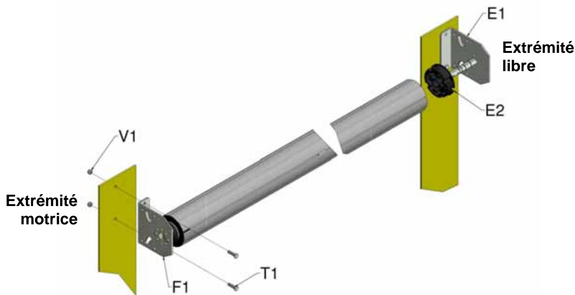
Figure 7a, Montage de portes jusqu'à 5 m de large au bâtiment
