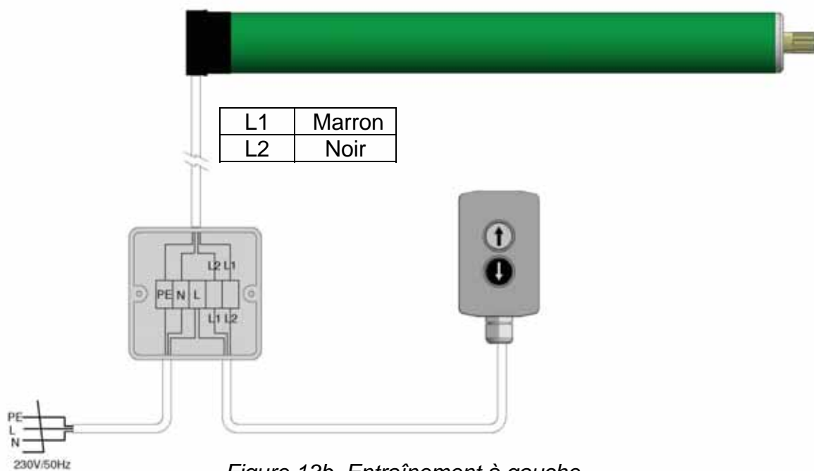
Figure 13b, Entraînement à gauche
