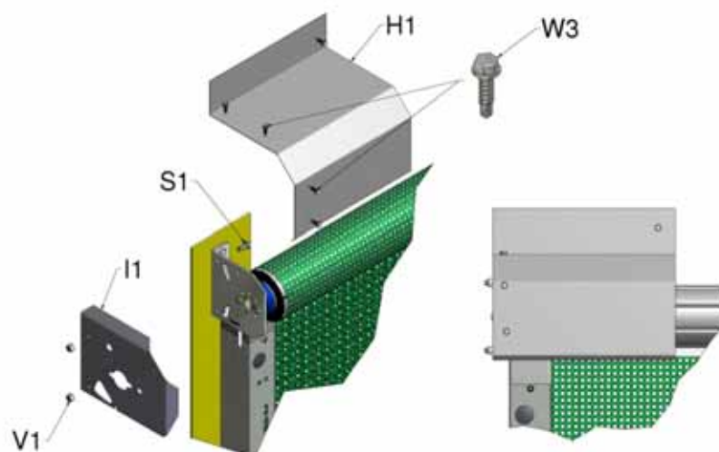
Afbeelding 18, Motorkapmontage
